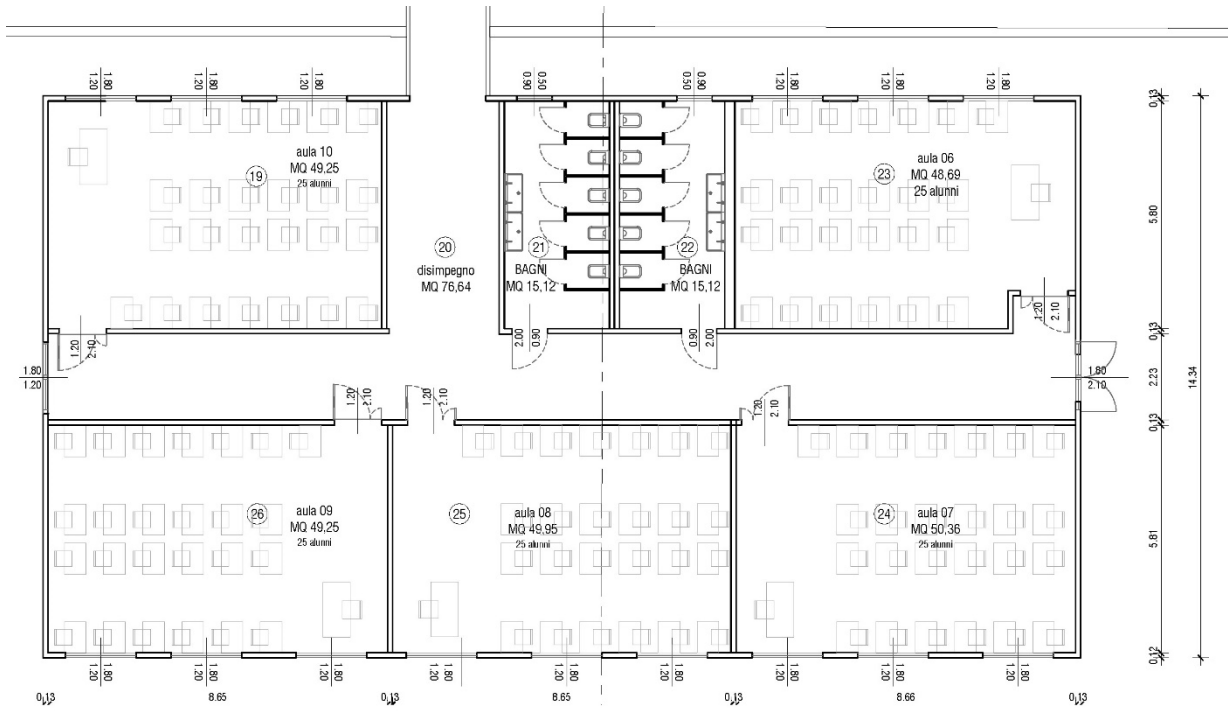
PIANO TERRA - PREFABBRICATO
